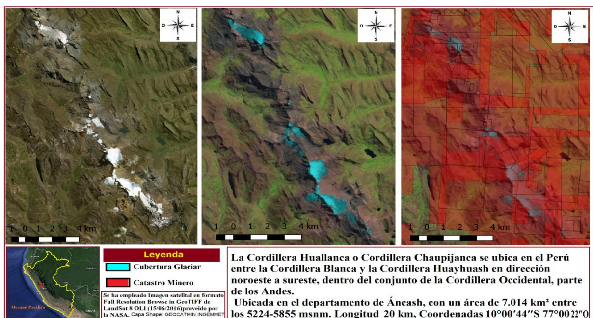
Figura 1.- Nevado Huallanca y unión de capas con catastro minero sobre glaciares.
