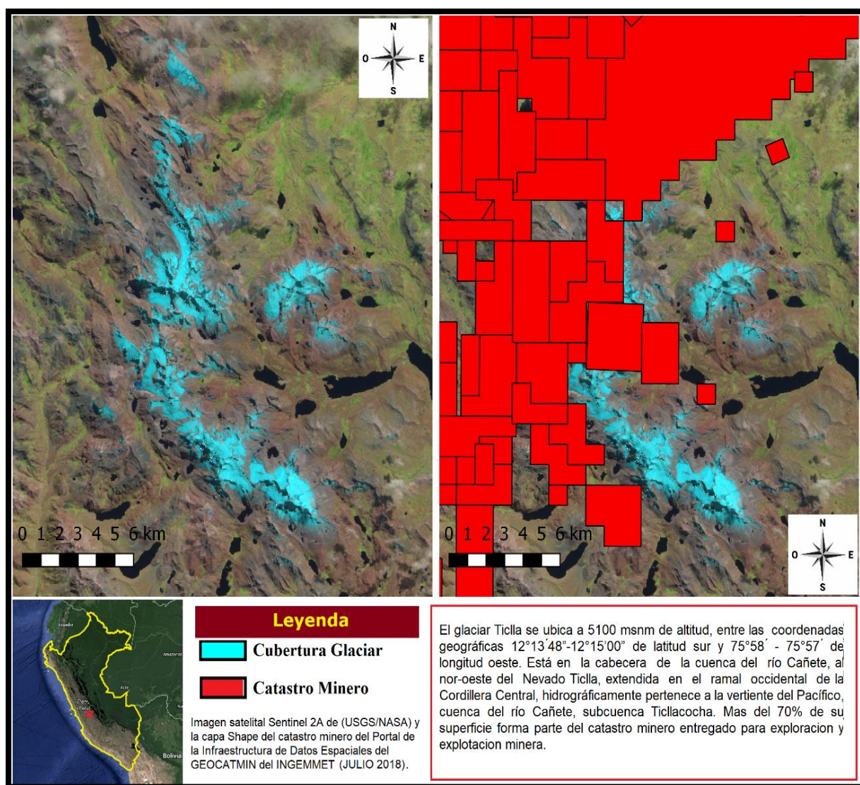
Figura 3. Nevado Ticlla y unión de capas con catastro minero sobre glaciares.
